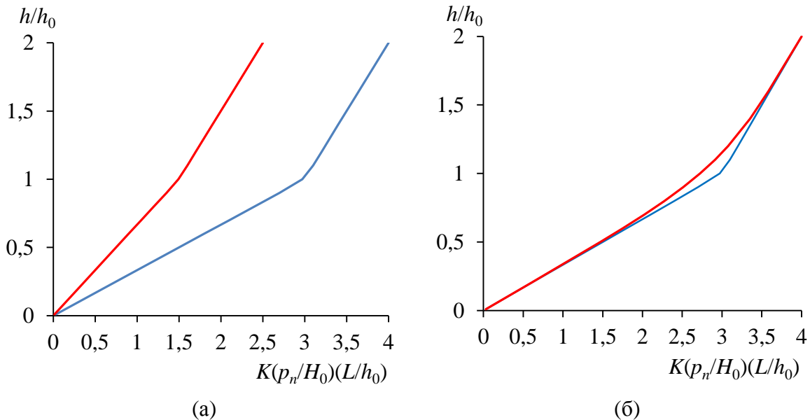
Рис. 3. Зависимость относительной величины линейного износа от безразмерного пути трения: влияние степени упрочнения \psi (верхняя кривая для \psi = 3 , нижняя – \psi = 1,5 ) (а); влияние параметра h_m (верхняя кривая для h_m/h_0 = 0,2 , нижняя – h_m/h_0 = 0,02 ) (б)
