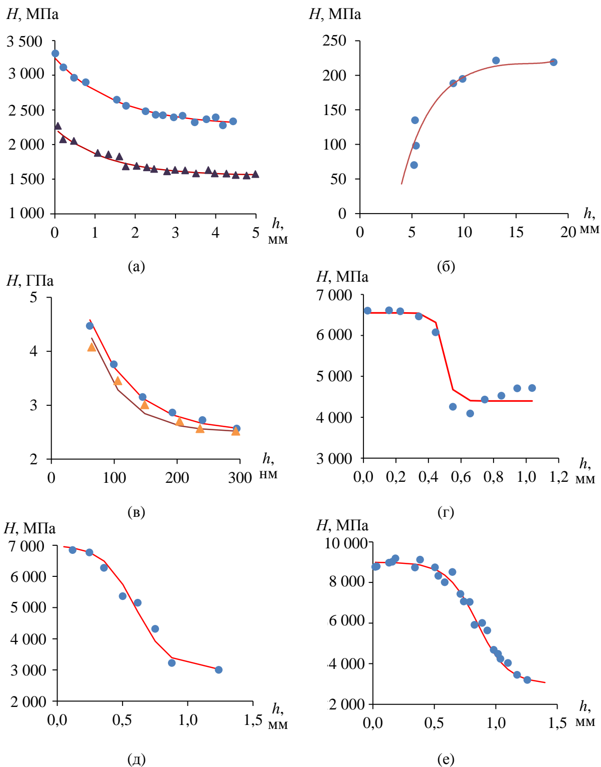
Рис. 2. Изменение твердости по глубине в зависимости от материала и технологии обработки поверхности: обкатка роликом (верхняя кривая – сталь 45Г2, нижняя – сталь 20) [19] (а); микротвердость, Cd [20] (б); нанотвердость, Ni, полировка (верхняя кривая – размер абразивного зерна 0,05 мкм, нижняя – 5 мкм) [21] (в); микротвердость, сталь 30ХГСА, лазерная закалка [22] (г); твердость по Кнупу, чугун, лазерное упрочнение [23] (д); твердость по Виккерсу, сталь 45, электронно-лучевая обработка [23] (е); точки – экспериментальные значения; линии – теоретические зависимости (см. уравнения (4) и (5))
