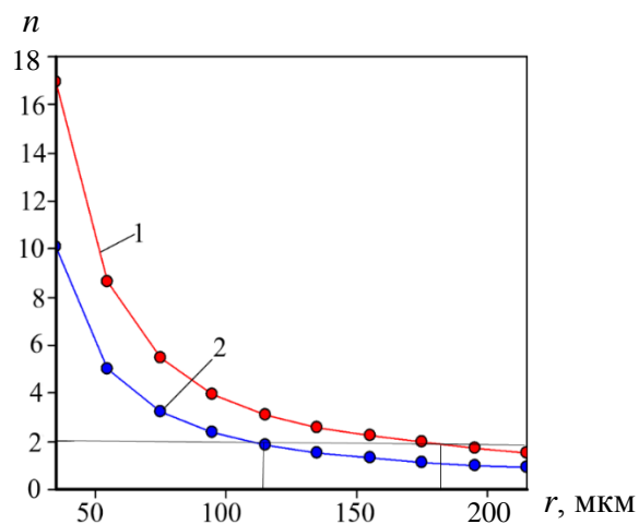
Рис. 6. Зависимость коэффициентов запаса n от радиуса скругления r режущей кромки: 1 – по пределу прочности; 2 – по пределу текучести
