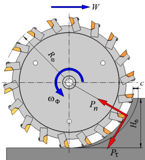
Рис. 1. Силы, действующие на режущий элемент фрезы
