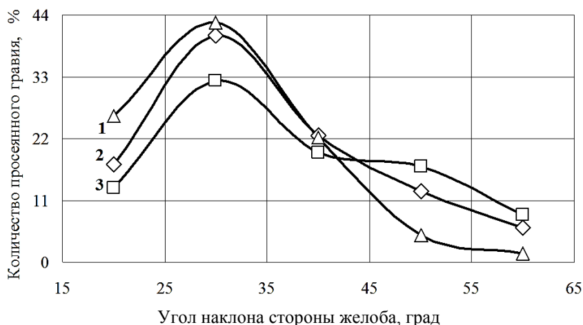
Рис. 7. Зависимость просеивания гравия по ширине желоба при частоте вращения валов с дисками, об/мин: 1 – 70; 2 – 105; 3 – 141
