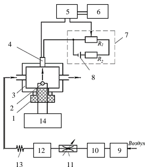
Рис. 1. Схема экспериментальной установки для исследований ИКППД:
