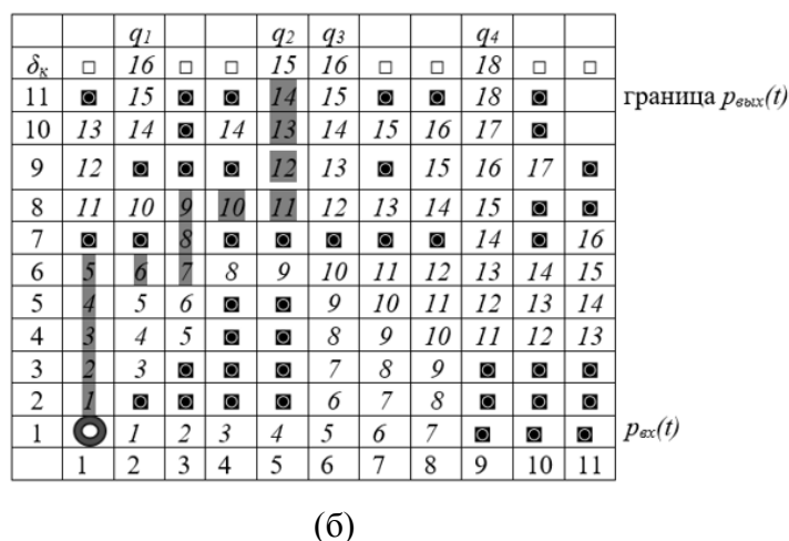
Рис. 2. Модель региона r_t в виде ДРП: граница выхода из региона (а); выбранный маршрут и выходная позиция q_2 (б)
