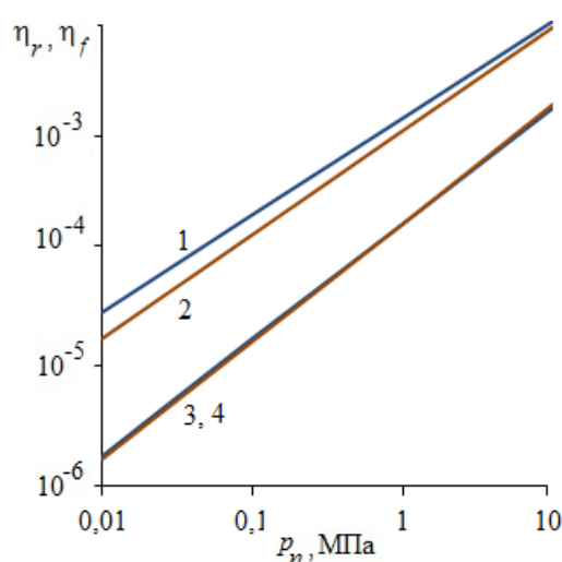
Рис. 4. Зависимости относительных фактической \eta_r (1, 2) и физической \eta_f (3, 4) площадей контакта от номинального давления; линии 1, 3 – v = 2 ; линии 2, 4 – v = 3
